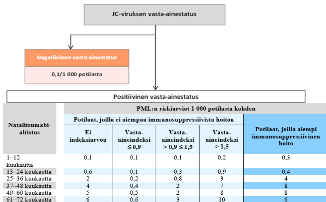
Kuva 1: PML:n riskiarvioalgoritmi
